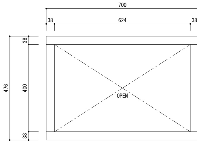
■正面图
