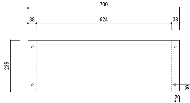
■平面图
