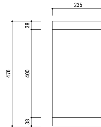
■侧面图
